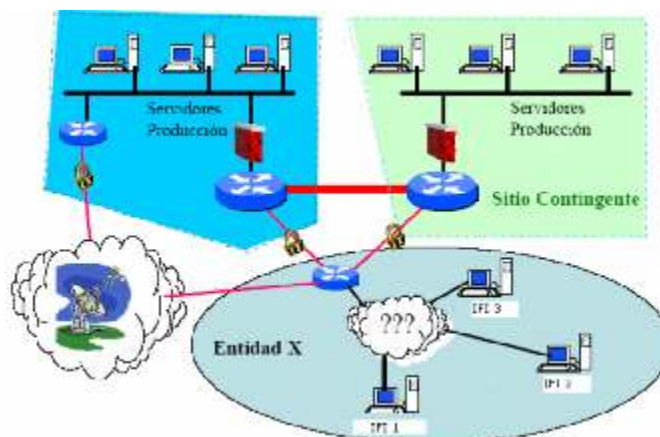
DIAGRAMA SIMPLIFICADO DE LA INFRAESTRUCTURA TECNOLÓGICA PROYECTADA PARA LA AGENCIA FINANCIERA DE DESARROLLO.
